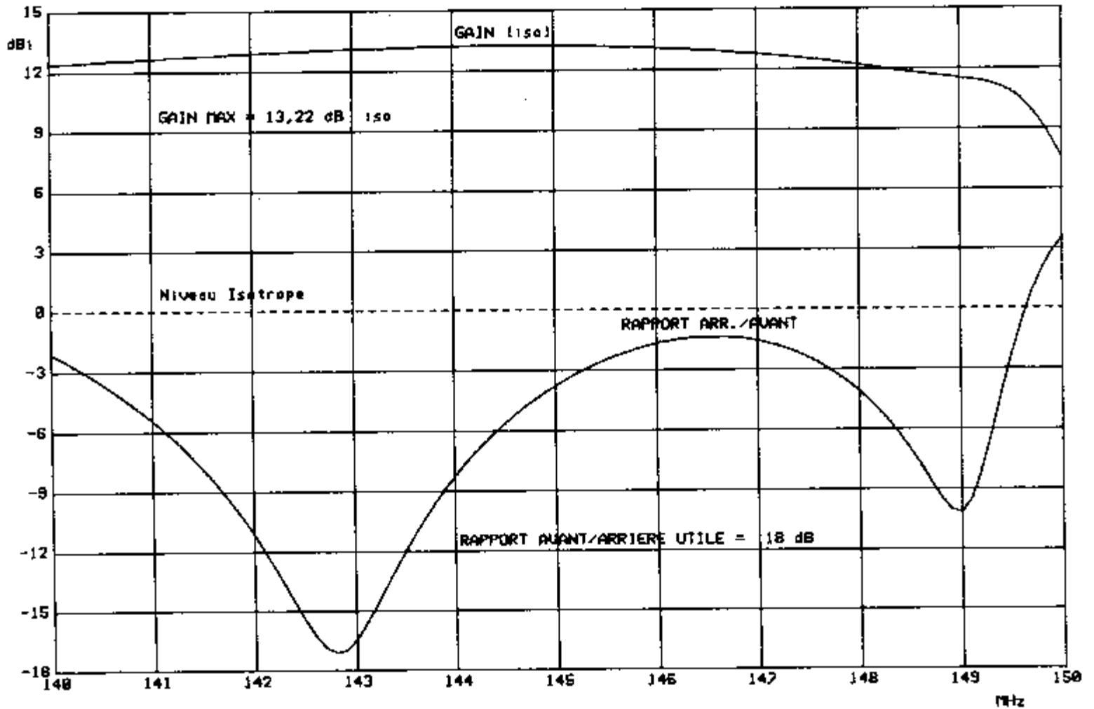
ANTENNE 9 ou 2x9 ELEMENTS YAGI: BANDE 144 - 146 MHz
